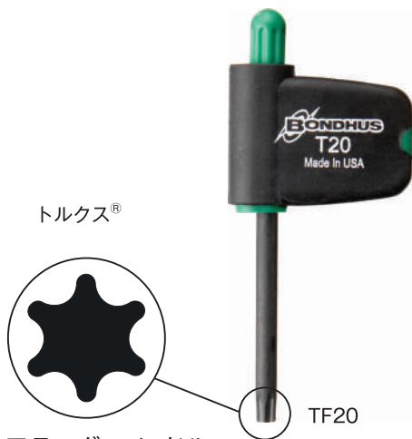
トルクス® フラッグ・ハンドル
